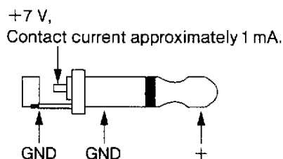
Plug wiring
